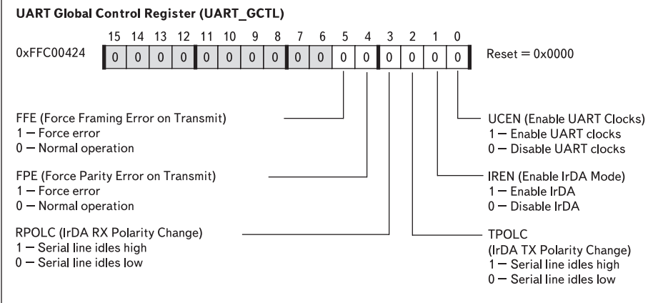
Рис. 2. Регистр UART Global Control Register (UART_GCTL)
