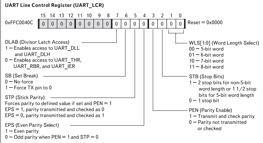
Рис. 3. Регистр UART Line Control Register
